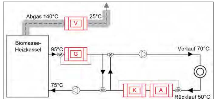
Abb. 2: Wärmefluss und Hauptkomponenten (Verdampfer V, Kondensator K, Absorber A und Austreiber/Generator G) der Sorptionswärmepumpe (links) und Einbindung der Absorptionswärmepumpe in das Wärmenetz des Biomassekessels (rechts).
