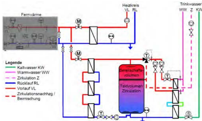
Bild 2: Vereinfachtes Funktionsschema der patentierten Fernwärmeübergabestation
