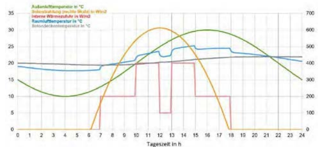
Temperaturverläufe als Ergebnis einer thermischen Gebäude- und Anlagensimulation
