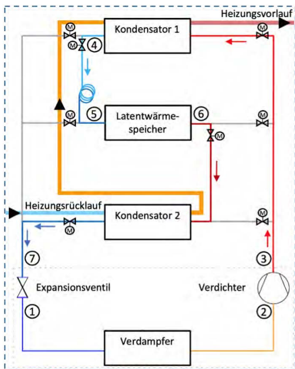
Abb. 4: Fließbild der Wärmepumpe mit integriertem Latentwärmespeicher, im Entladebetrieb mit serielltem Durchgang des Kältemittels durch Kondensator 1, Latentwärmespeicher und Kondensator 2 (links). Versuchsanlage (rechts) mit internem Wärmepumpenkreislauf (linke Frontseite) und Latentwärmespeicher (rechter Anlagenteil).
