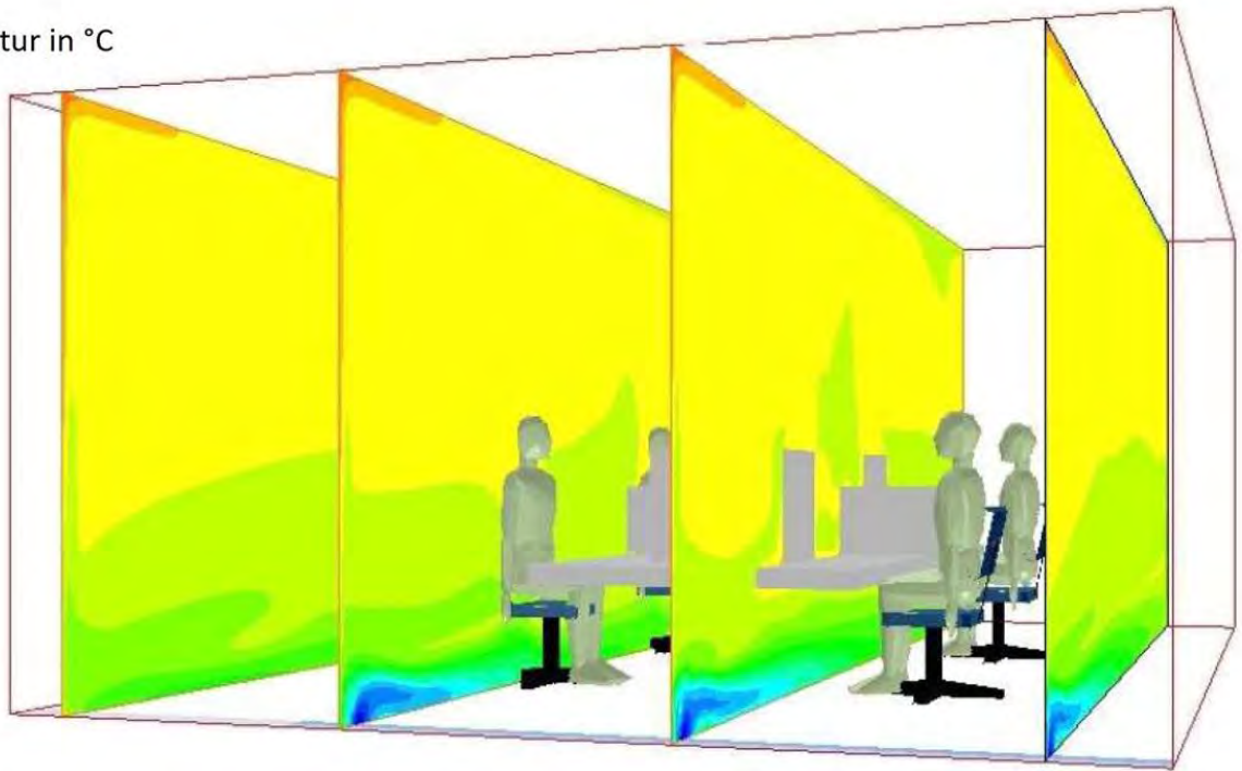
Temperaturverteilung im Raum als Ergebnis einer Raumluft-Strömungssimulation (CFD)
