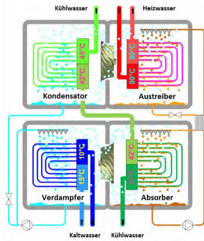
Abb. 1: Fließbild der Absorptions-/Kompressions-Kältemaschine mit Turboverdichter zwischen Verdampfer und Absorber oder Austreiber und Kondensator. Einsatz für 10 °C Kaltwassererzeugung mit Rückkühlung durch ein trockenes Rückkühlwerk mit Kühlwasservor-/ -rücklauf 37/45 °C. (links). Funktionsmuster der Hybridkälteanlage mit wissenschaftlicher Messtechnik in der Hardware-in-the-Loop-Teststandumgebung im Labor der Hochschule München (rechts)
