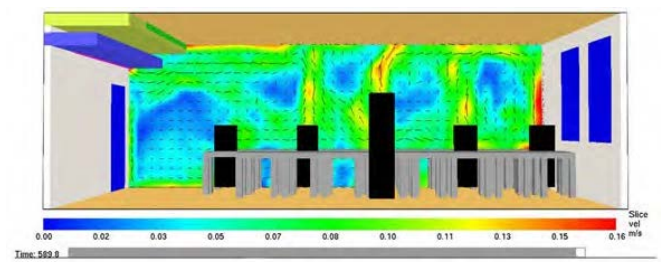
Abbildung 1: Luftdurchströmung im Hörsaal G3.30
