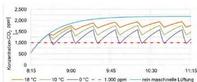
Abbildung 2: \text{CO}_2 -Konzentration im Hörsaal G3.30 bei hybrider Lüftung mit 18^\circ\text{C} , 10^\circ\text{C} und 0^\circ\text{C} Außentemperatur, Eigene Auswertung der Simulation nach einem Tool von IBO Innenraumanalytik OG (2017)
