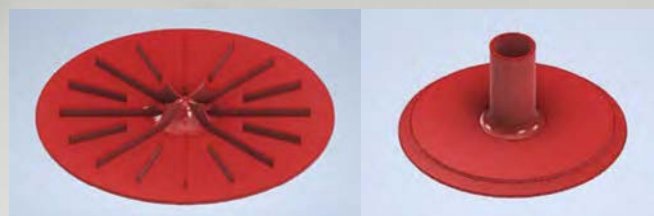
Abb. 2: Radialdiffusor als Schichtladeeinrichtung in einem thermischen Speicher (3D-Druck)
