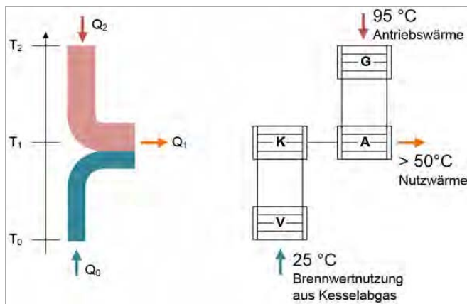
Abb. 2: Wärmefluss und Hauptkomponenten (Verdampfer V, Kondensator K, Absorber A und Austreiber/Generator G) der Sorptionswärmepumpe (links) und Einbindung der Absorptionswärmepumpe in das Wärmenetz des Biomassekessels (rechts).
