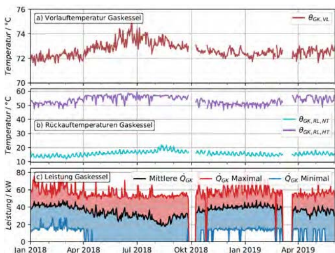
Bild 3: Messergebnisse einer GEWOFAG-Wohnanlage: Erdgas-Brennwertkessel mit zwei Rücklaufanschlüssen und hocheffizienter TWE mit kontinuierlich niedrigen Rücklauftemperaturen ( \theta_{GK} , RL, NT) meist unter 20 °C
